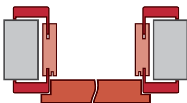
nákres falcových dveří
